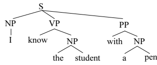
図2 構文解析結果 Fig. 2 Parse tree.
