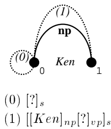
図 2: 語“Ken”が入力された時点でのチャート
