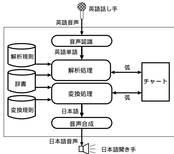
図 1: 漸進的な英日話し言葉翻訳システムの構成
