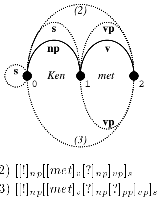
図 3: 語“met”が入力された時点でのチャート
